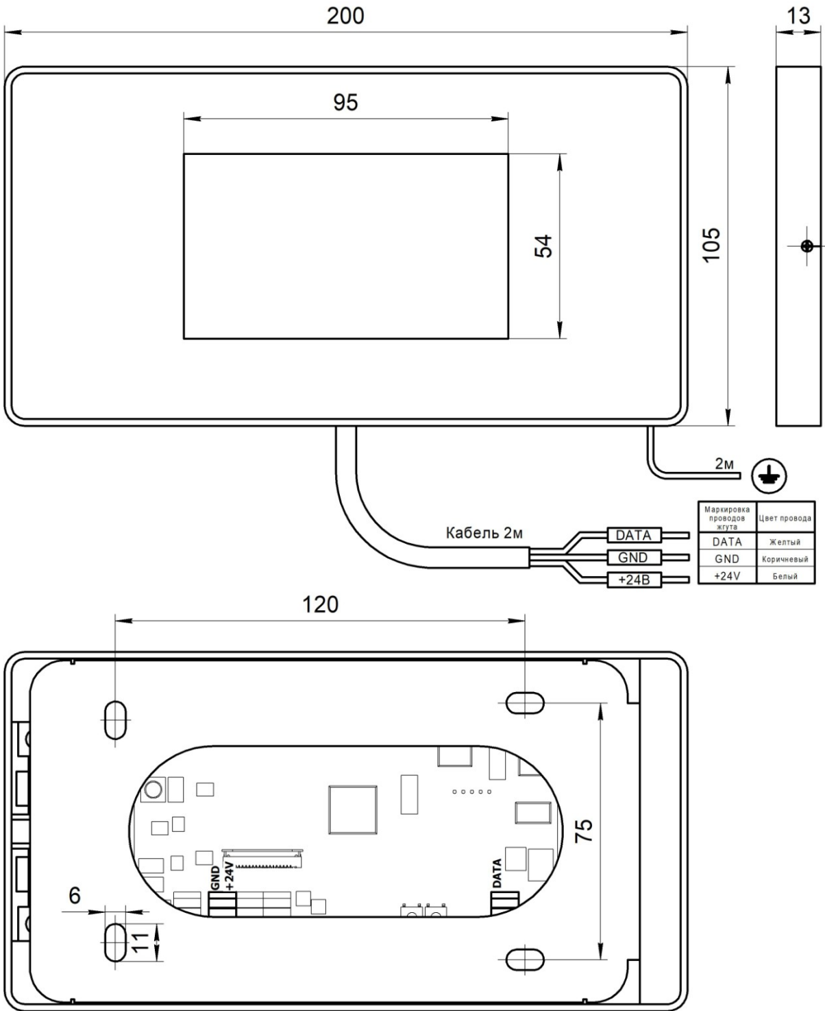
Рис.1 Внешний вид Табло накладное МАЛАХИТ НШЕК.468232.127-01 (дисплей 4,3)
